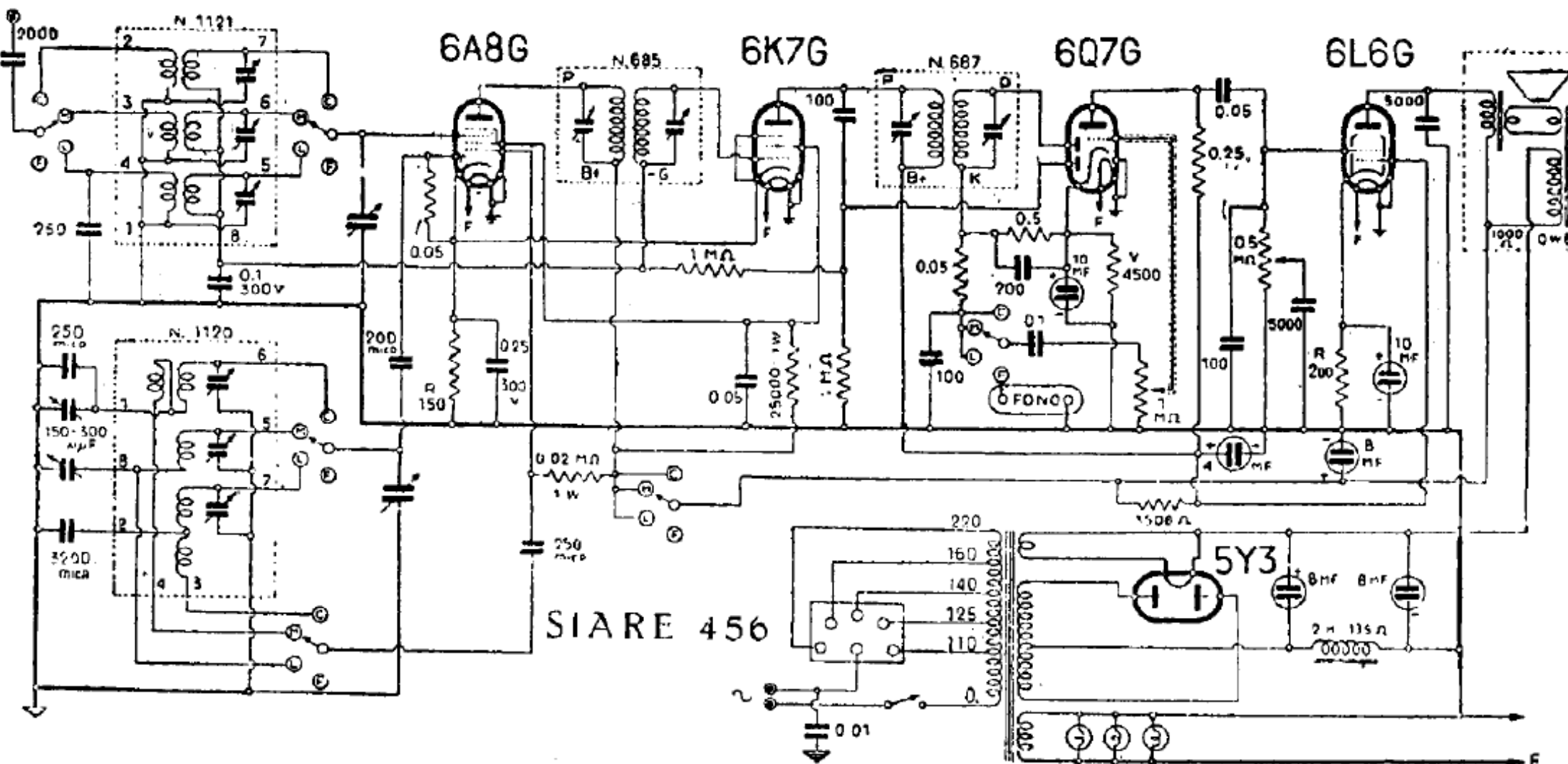
RADIO SIARE. — Mod. « 456 » e « Crosley 255 ». — Produzione 1938-39. — Media frequenza: 487 kHz.
